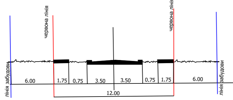
Поперечний профіль вулиці Зацепи
