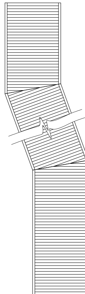
Деталь 4. Принцип стикування дощатого настилу на вигинах стежки
