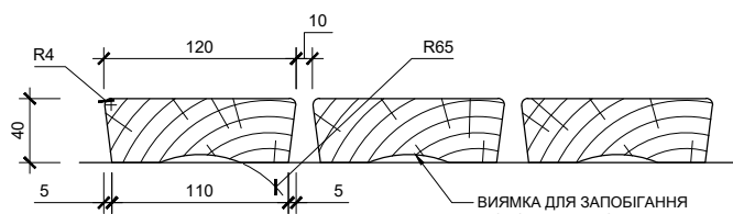
Деталь 3. Профіль дощатого настилу
