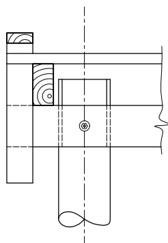
Деталь 2. Кріплення балок до опор
