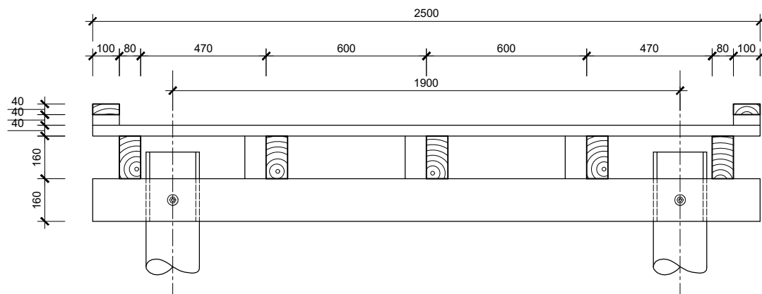
Деталь 1. Несуча конструкція дощатого настилу
